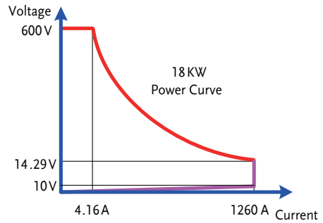
PEL-5018C-600-1260
