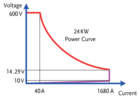
PEL-5024C-600-1680
