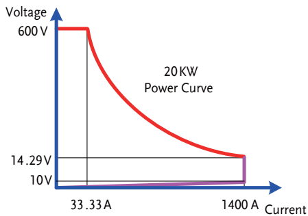
PEL-5020C-600-1400
